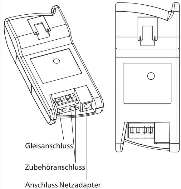
Abb. 2 – Das Regelgerät von unten mit Anschlusskennzeichnung
